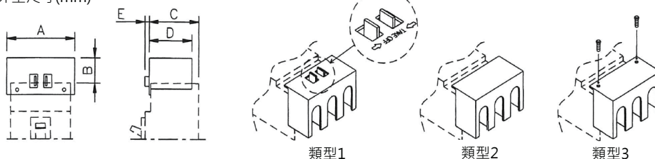
保護蓋類型--外型尺寸(mm)
